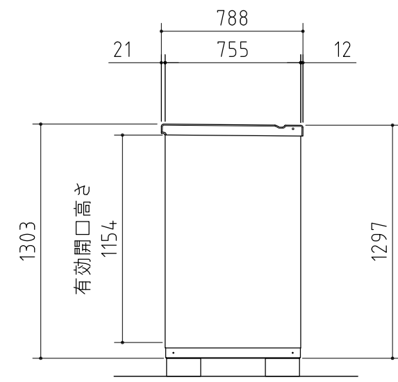
側面図
