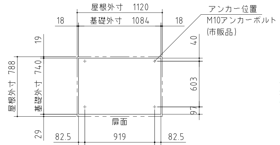
ベタ基礎図
